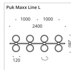
Kabellänge für Abhängung 2.000 mm (kürzbar) Cable length for suspension 2.000 mm (can be shortened)
